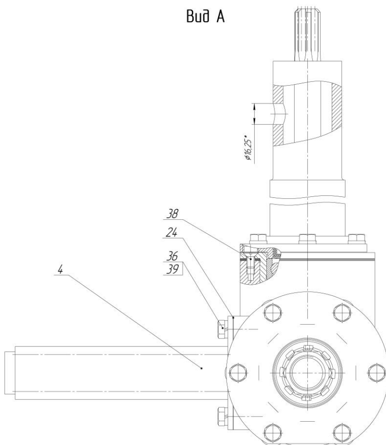
Рисунок 2 – Редуктор ФР-00.840
