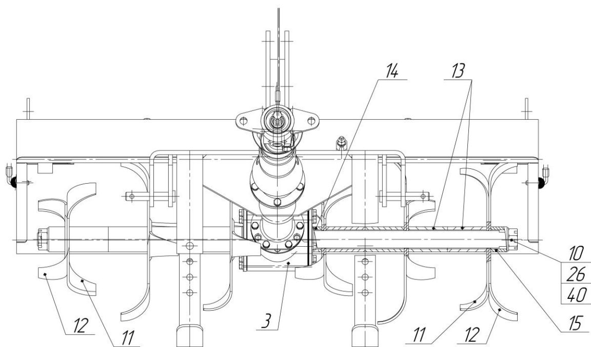
Рисунок 1 – Фреза почвообрабатывающая ФР-00.700-Б
